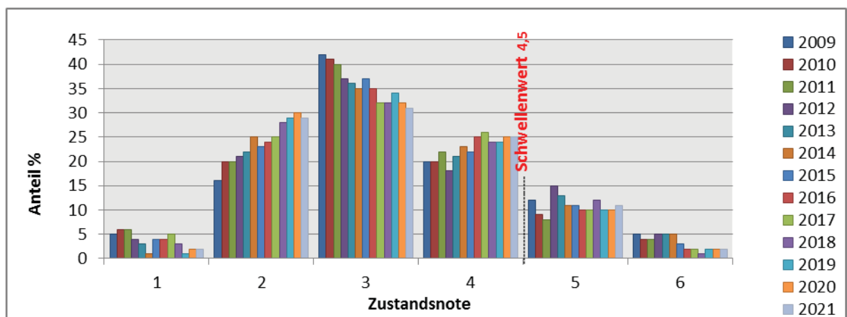
Abb. 4 Zustandsentwicklung (Trend)
