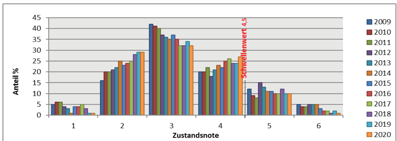
Abb. 4 Zustandsentwicklung (Trend)
