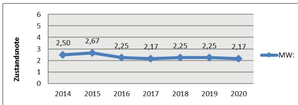
Abb. 8 Zustandsentwicklung Kreis-Brücken (Zustandsnote-Mittelwert)
